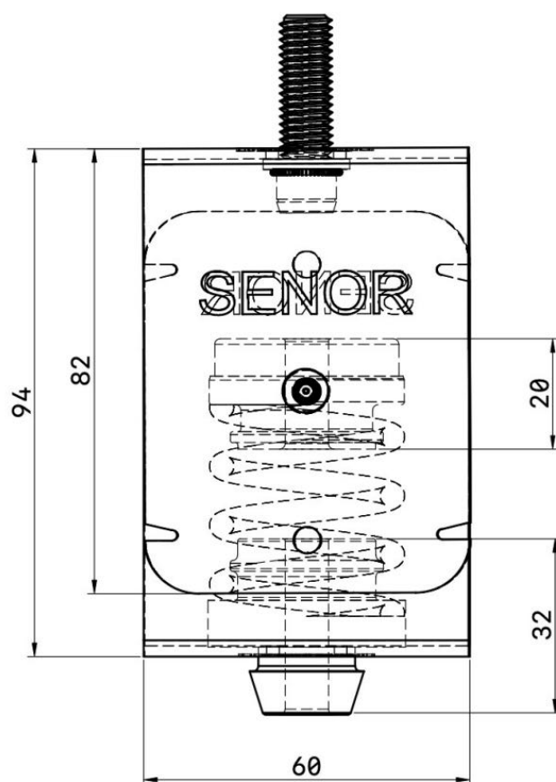
VISTA LATERAL
