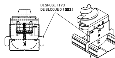
PERFIL DE TECHO. (F530, TC-47, MAESTRA 47/17 o SIMILAR)
