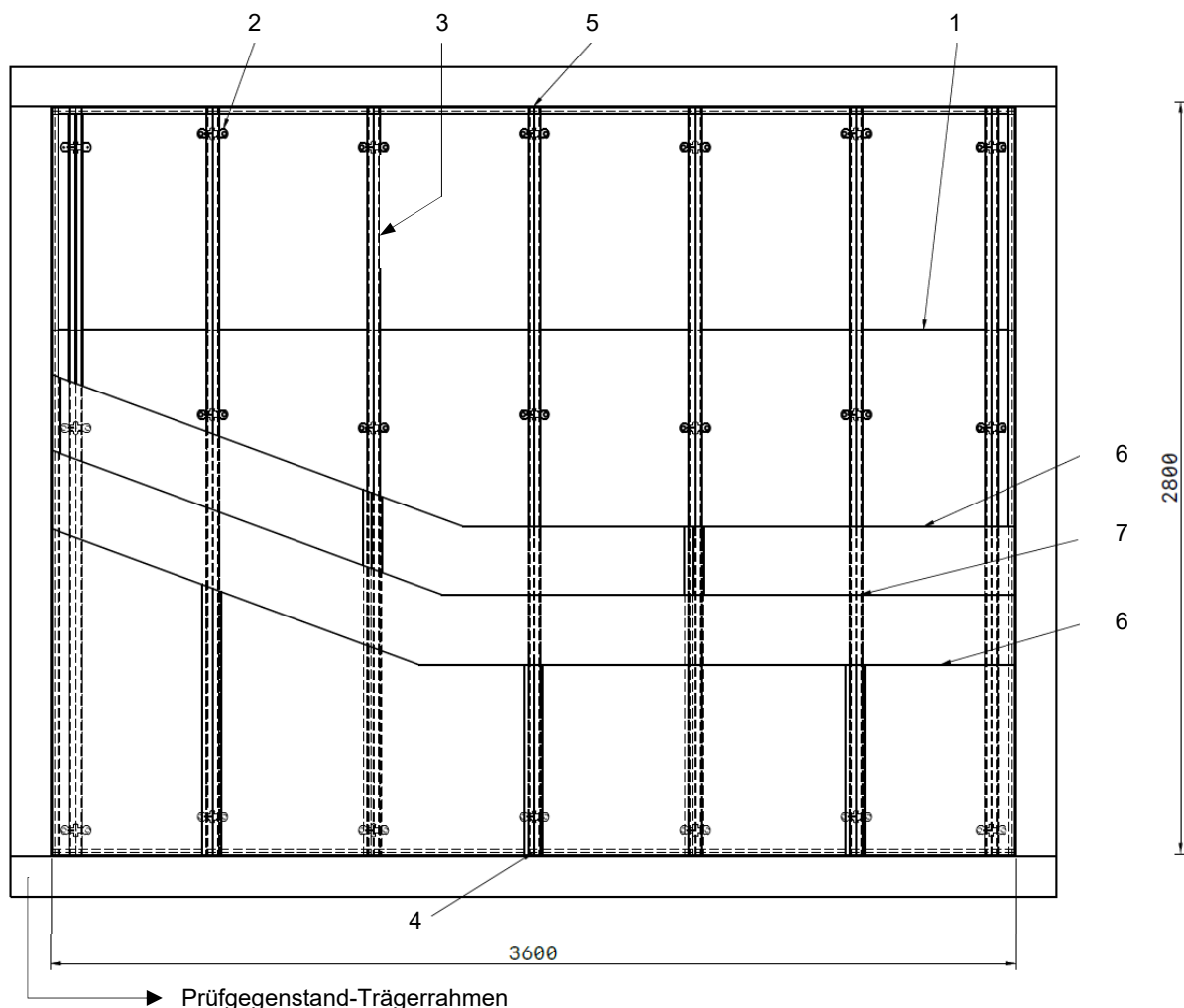
Schema 1 - Abmessungen in mm
