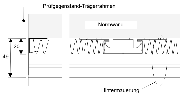
Schema 2 - Abmessungen in mm
