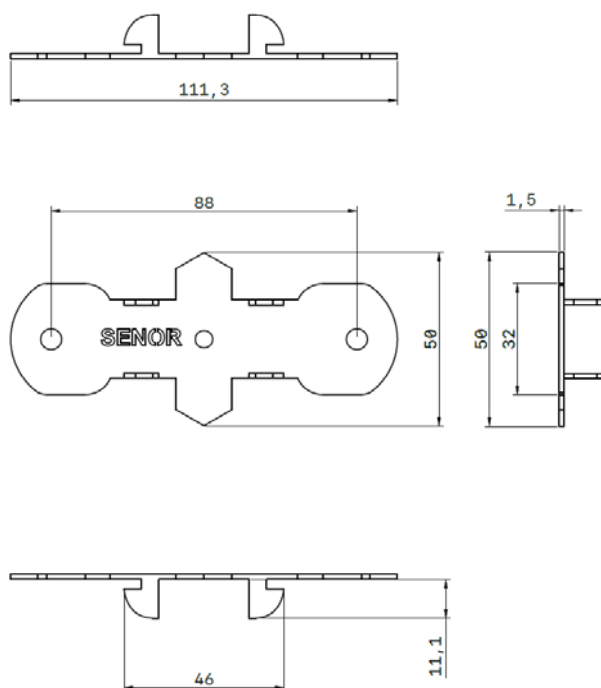
Schema 4 - Abmessungen in mm
