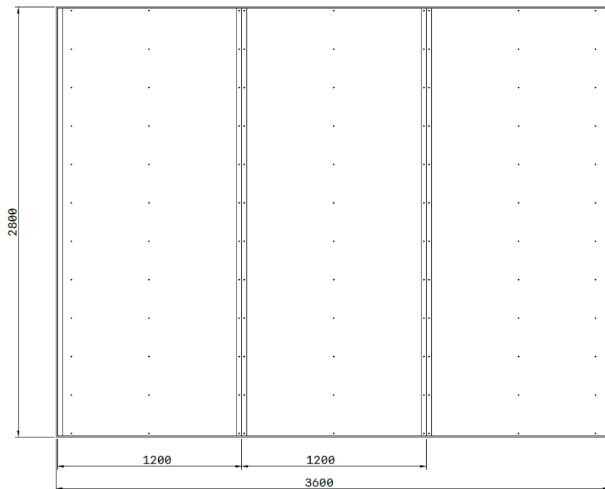
Schema 5 (Innenschicht) - Abmessungen in mm
