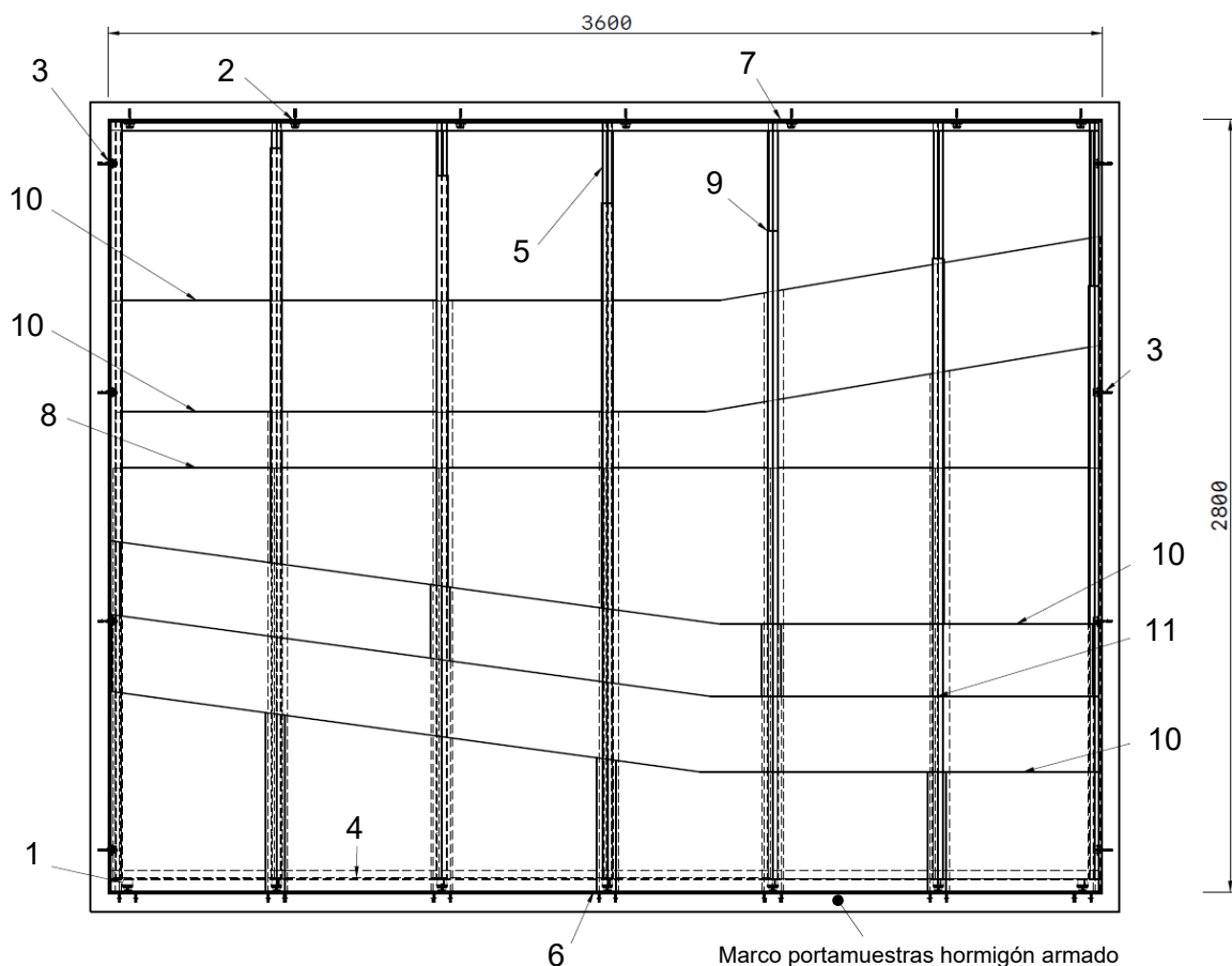
Esquema 1 - Alzado
