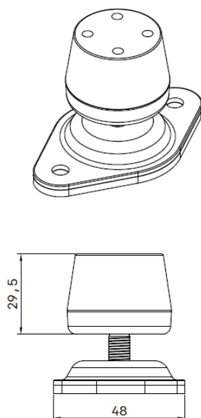
Tapones acústicos SE-TAV-500/11 R (rojo) y SE-TAV-500/11 A (azul)
