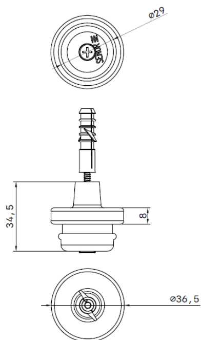
Tapones acústicos SE-TAV-500/11 R (rojo) y SE-TAV-500/11 A (azul)
