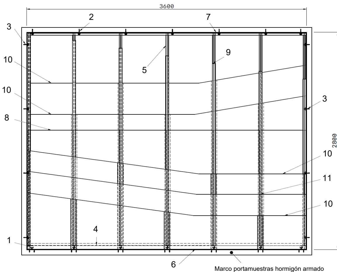
Esquema 1 - Alzado
