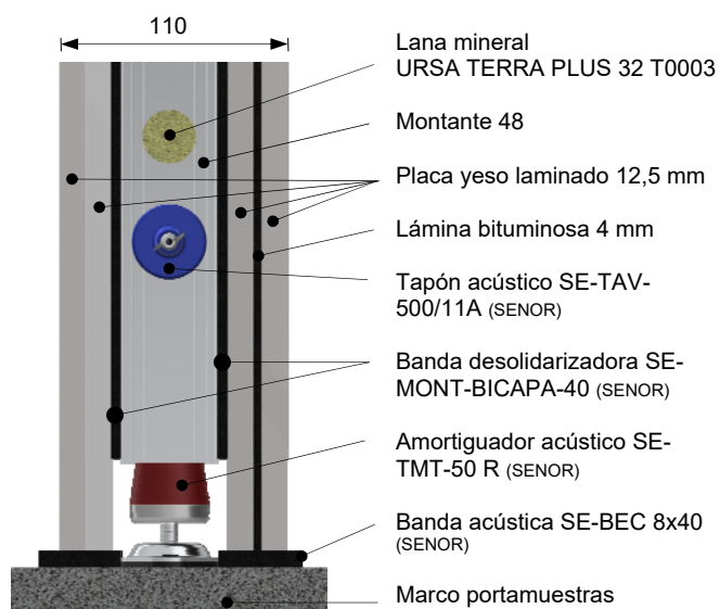
Esquema 2 - Sección vertical
