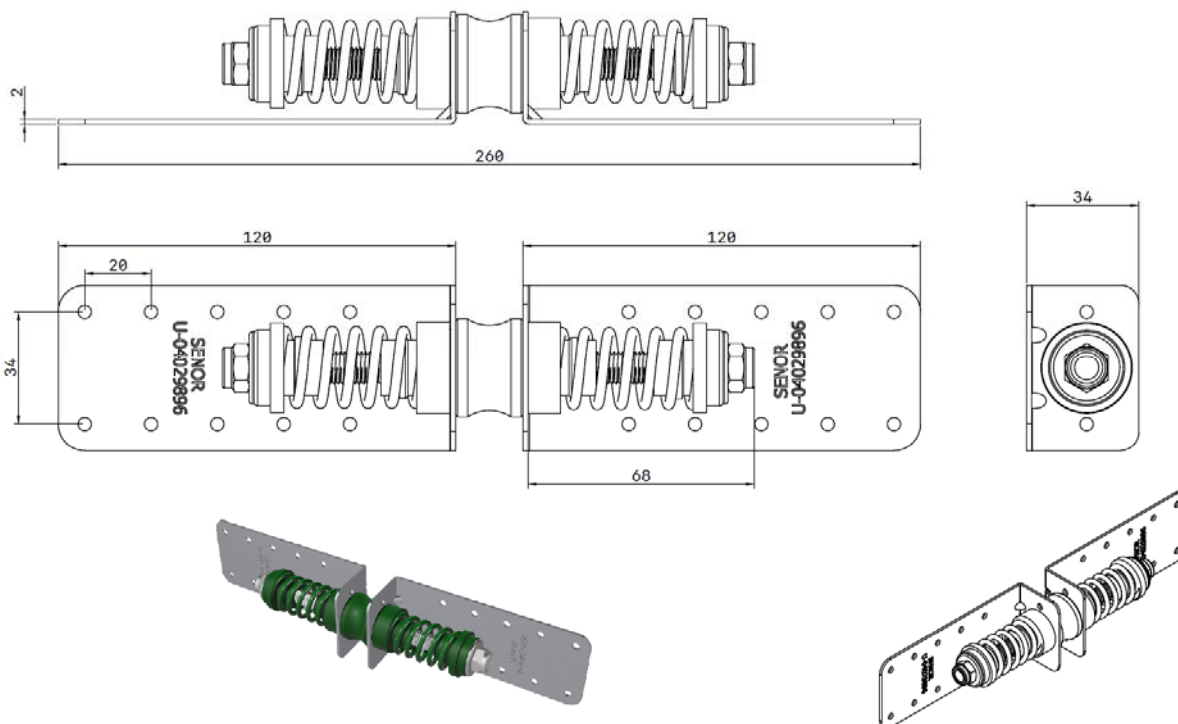
Amortiguador acústico SE-9600-TBM2
