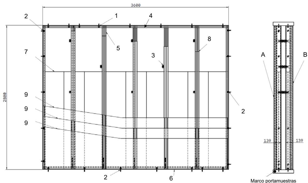
Esquema 1 - Alzado muestra. Cotas en mm
