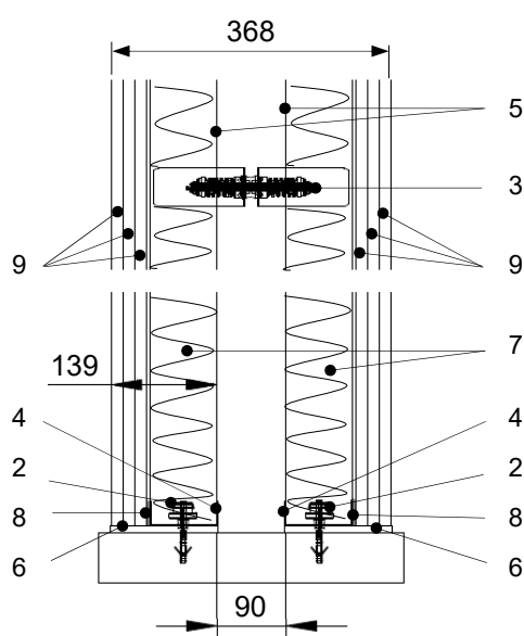
Esquema 2 – Sección vertical muestra. Cotas en mm
