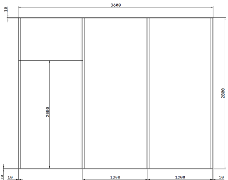
Esquema 5 – Disposición de placas yeso laminado cara A. Cotas en mm
