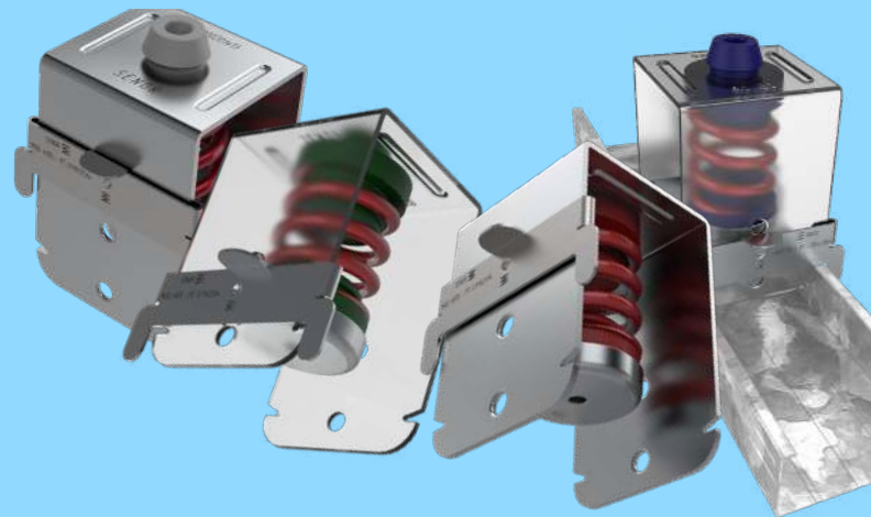
Mod. 60M/DS
