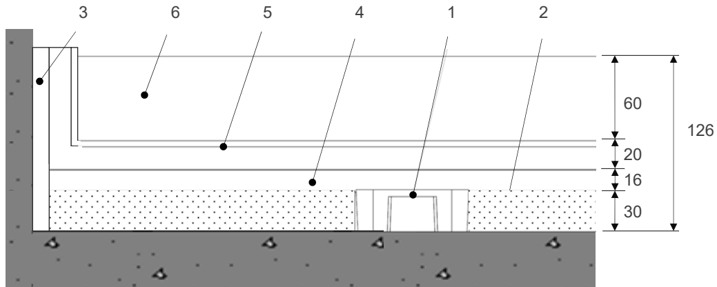
Schéma 1 – Section verticale. Mesures en mm
