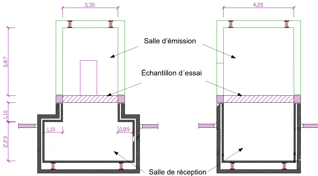
Schéma des salles acoustiques de transmission verticale
