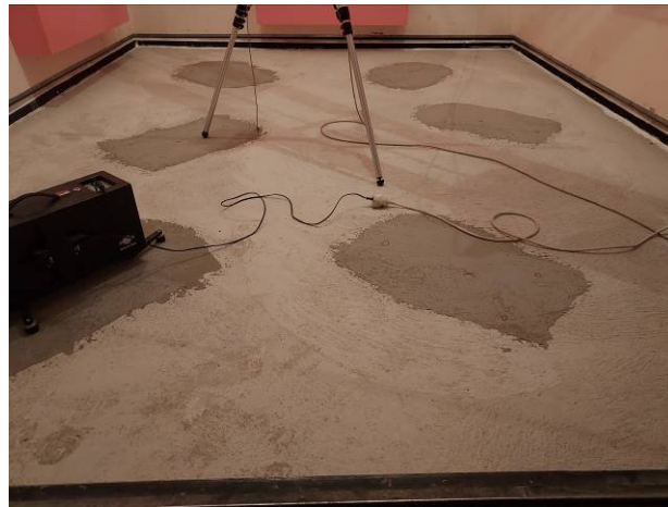
Photographie de l'échantillon d'essai dans les salles d'essai
