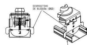
PERFIL DE TECHO. (F538, TC-47, MAESTRA 47/17 o SIMILAR)
